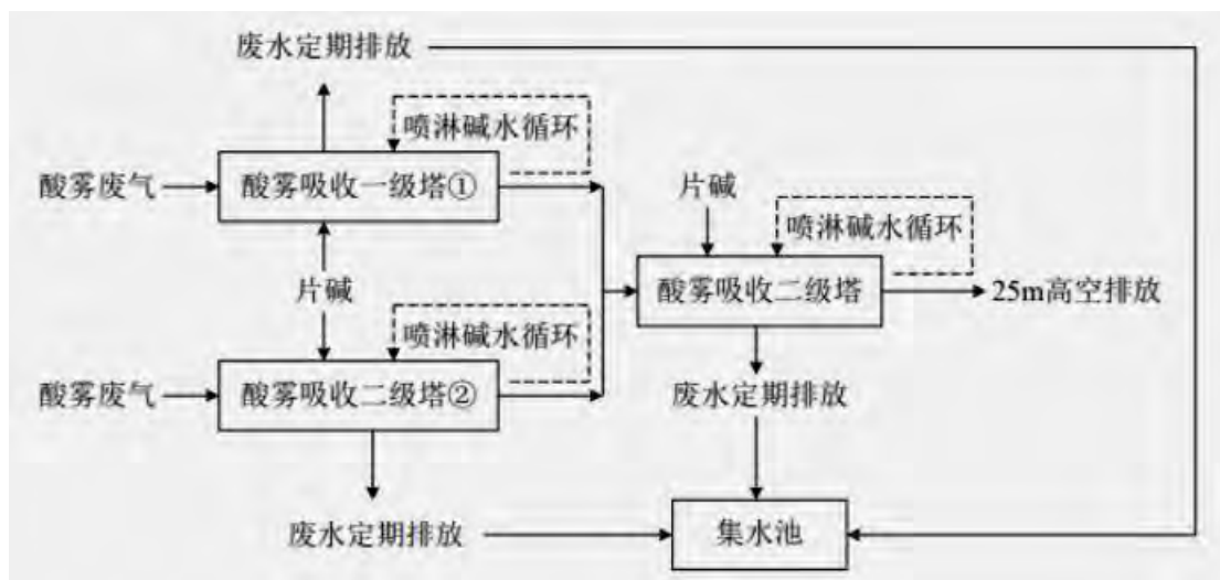
图4.1-8 废气处理工艺流程
