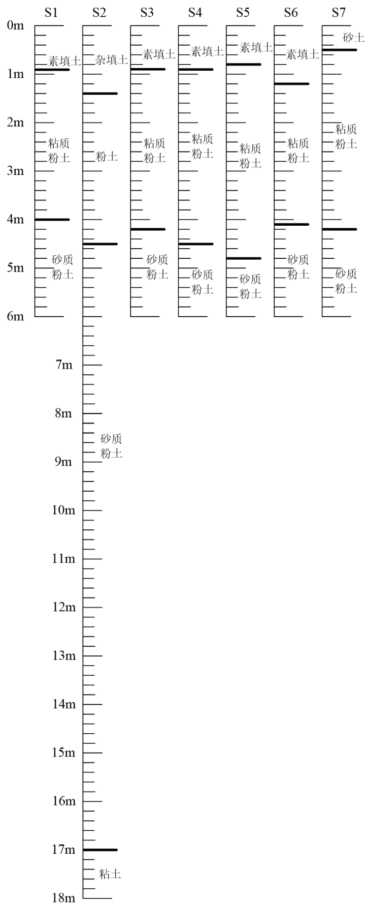
图6.1-1 土层分布截面图
