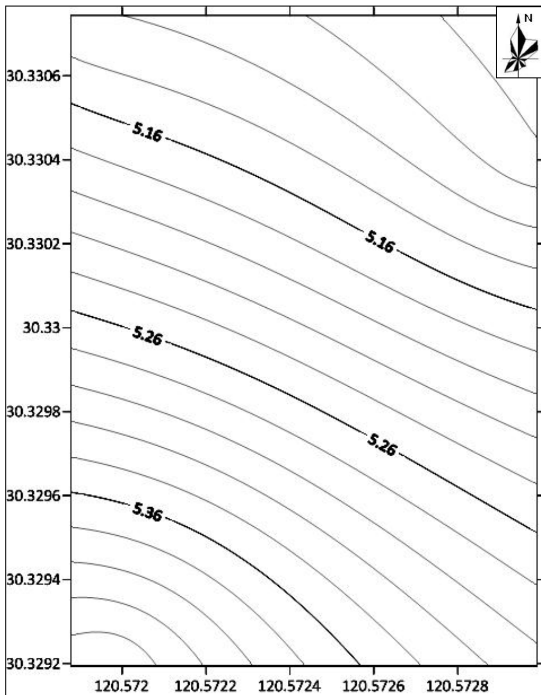
图 3.1-5 地块等水位线示意图
