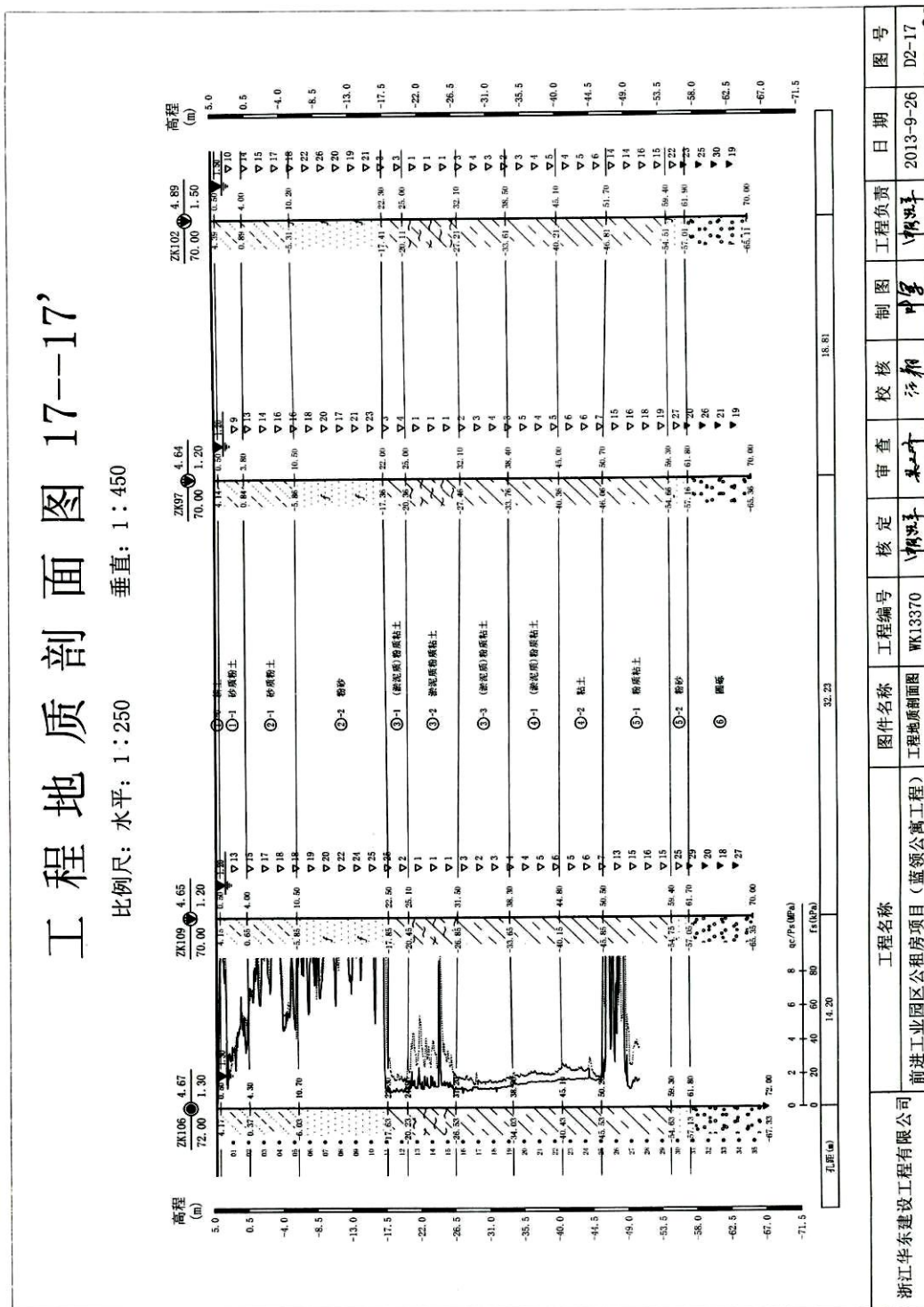
3.1-3 前进工业园区公租房项目（蓝领公寓工程）岩土工程地质剖面图
